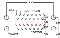
PCB布局 (PCB Layout)
